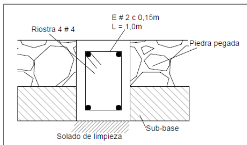
Corte Transversal Sección en Piedra Pegada
